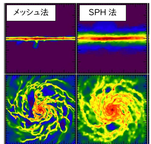
図1：数値コードによって物理が異なる図 [Kim et al. (2016)のFigure 2. より引用]
